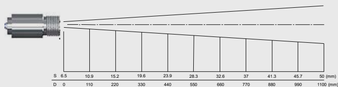
SF optics D:S = 22:1
